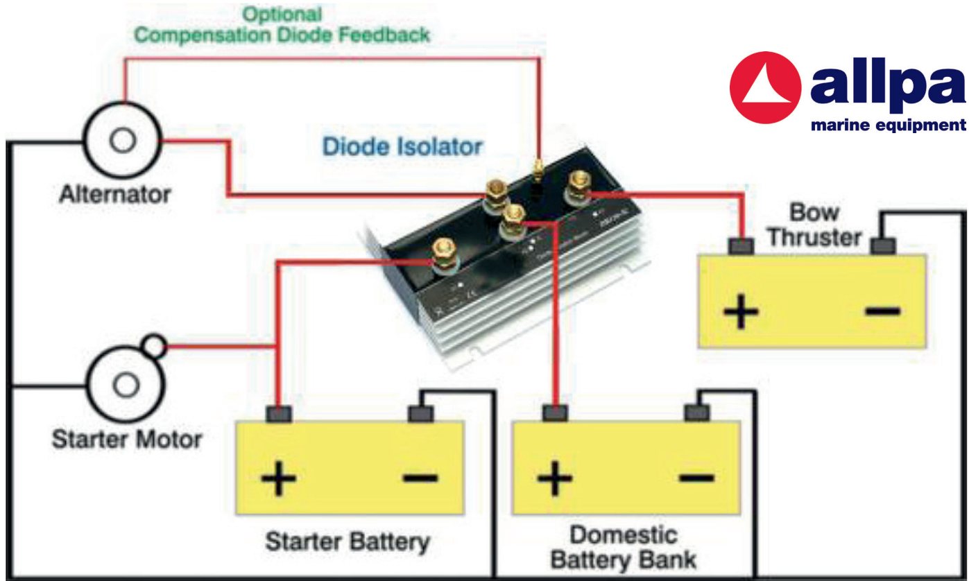
Schema DB 120-3C
